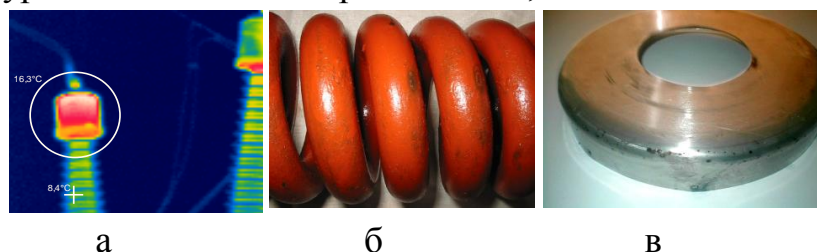
Рис. 2. Підвищений нагрів компенсаторів тиску вводів
