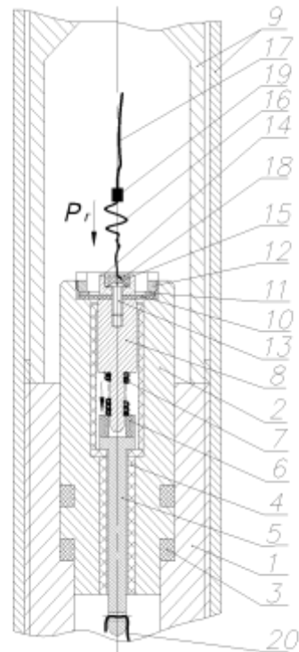
Рис. 2. Вдосконалений корпусний кумулятивний перфоратор (фрагмент) з електровводом нової конструкції:
