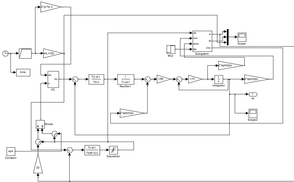
Рис. 11. Модель системи частотно-струмового управління з регулюванням спрямленого струму та швидкості
