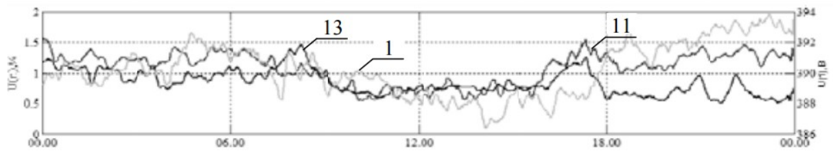
Рис. 3. Гармоніки напруги
